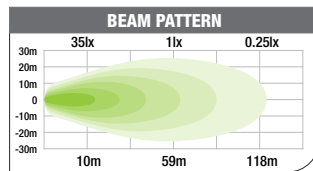
ILED5B
