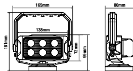
ILED5B
